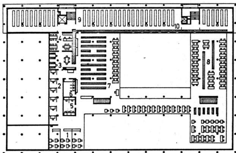
3. ábra A II. emelet alaprajza
