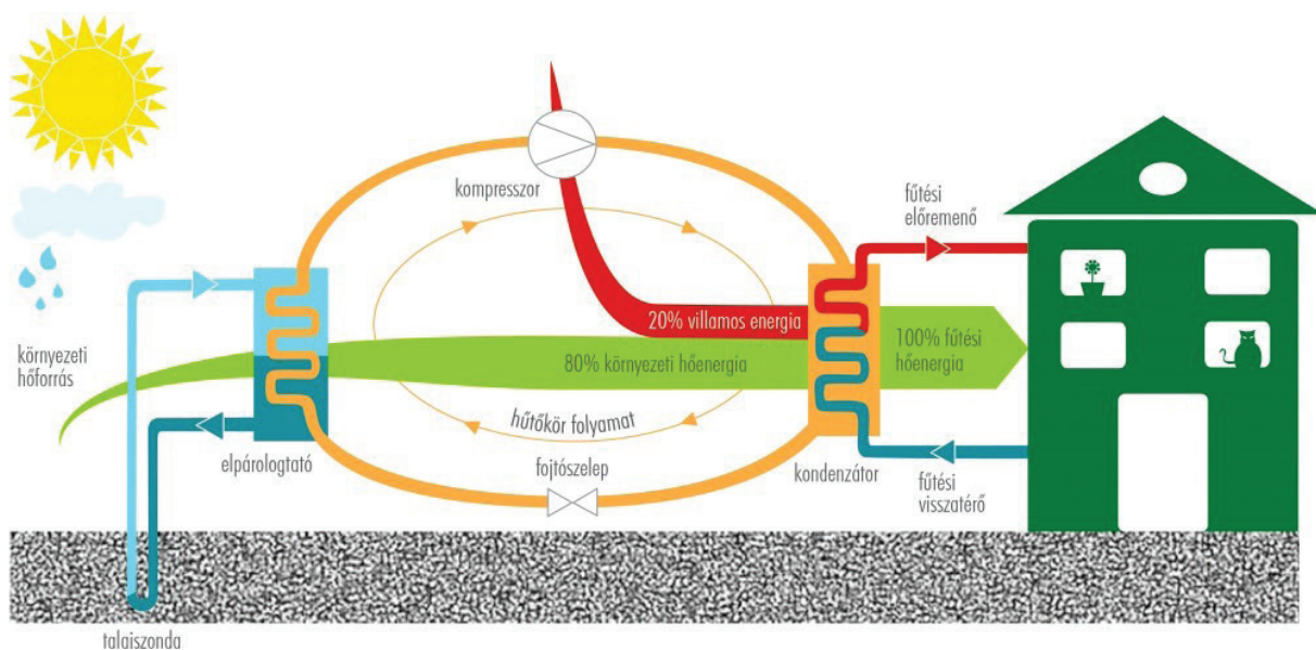
9. ábra A hőszivattyúk működési elve (forrás: https://www.oktoklima.hu )
